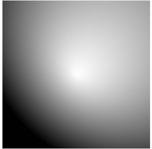
RadialGradient()
